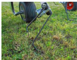
Das Futter wird ziehend mit dem 7,5 cm langen Haken am Fendt Performance Zinken aufgenommen.
